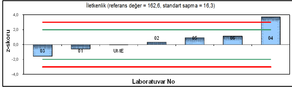
Şekil 1. Toprakta iletkenlik tayini z-skorumları
